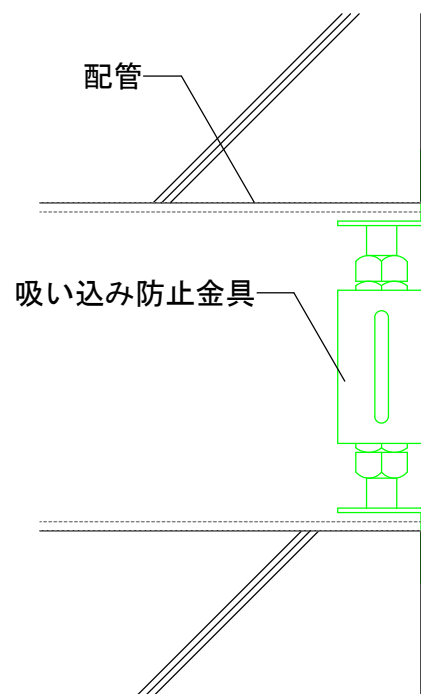
断面図
