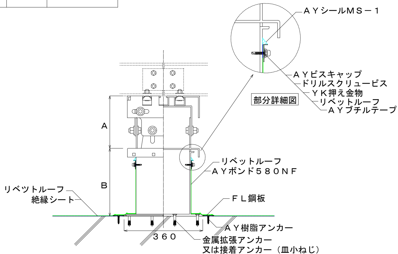
H鋼設置イメージ
