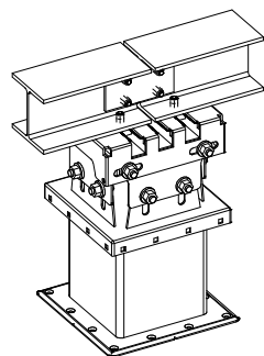
H鋼設置イメージ
