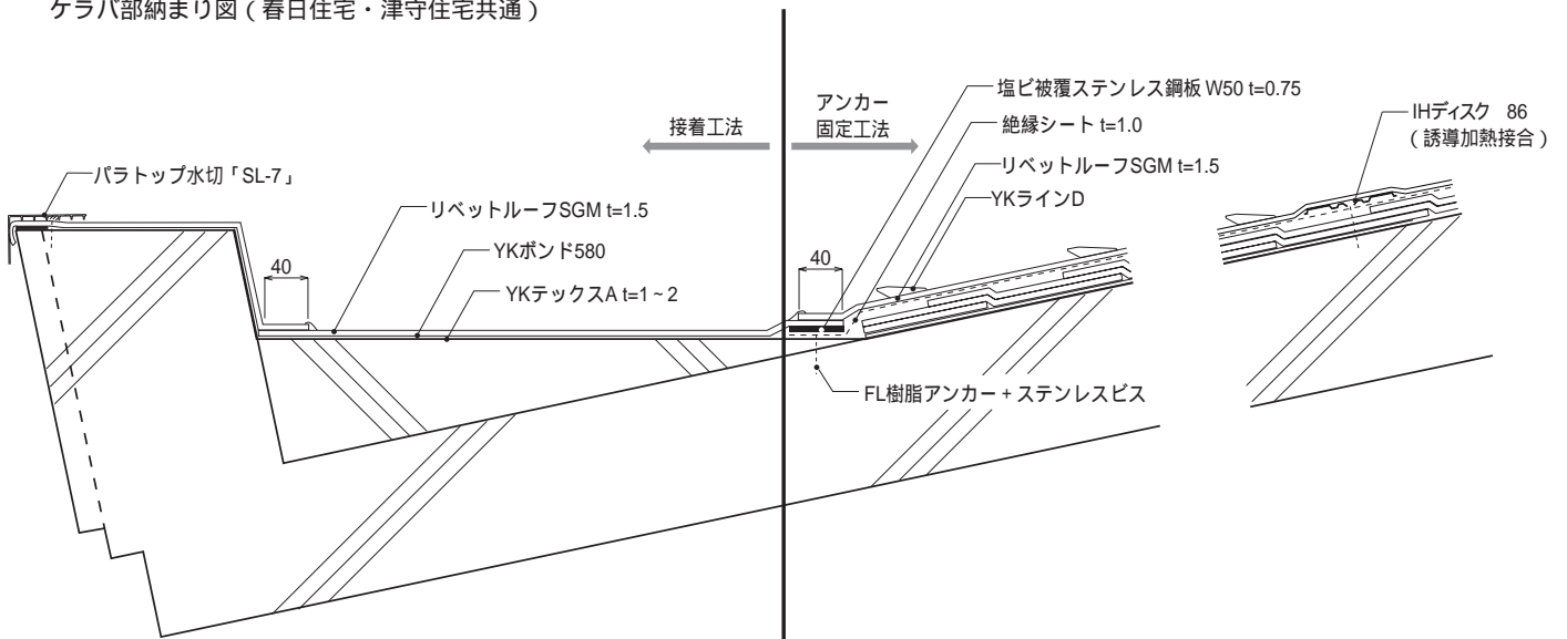
ケラバ部納まり図(春日住宅・津守住宅共通)
