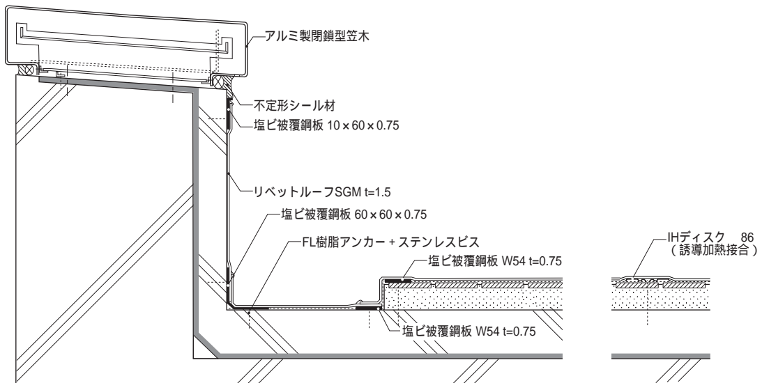
立上がり部納まり図
