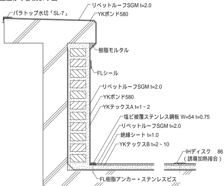
理学部A棟立上がり部納まり図
